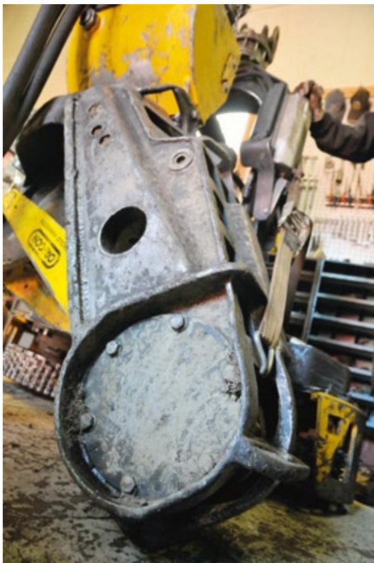
Bengt-Ola Börjesson har bland annat låtit flytta delar av arbetsbelysningen och förstärkt såglådan på aggregatet för att förbättra produktiviteten och hållbarheten.
